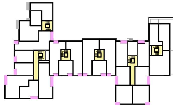
4NP +9,00 2445 m 2 HPP 101 m 2 lodžie 18 m 2 balkóny
