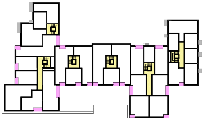
3NP +6,00 2575 m 2 HPP 97 m 2 lodžie 37 m 2 balkóny
