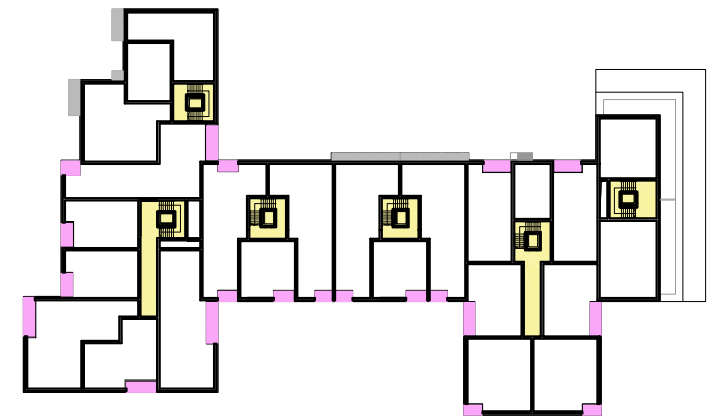
5NP +12,00 2320 m 2 HPP 101 m 2 lodžie 37 m 2 balkóny
